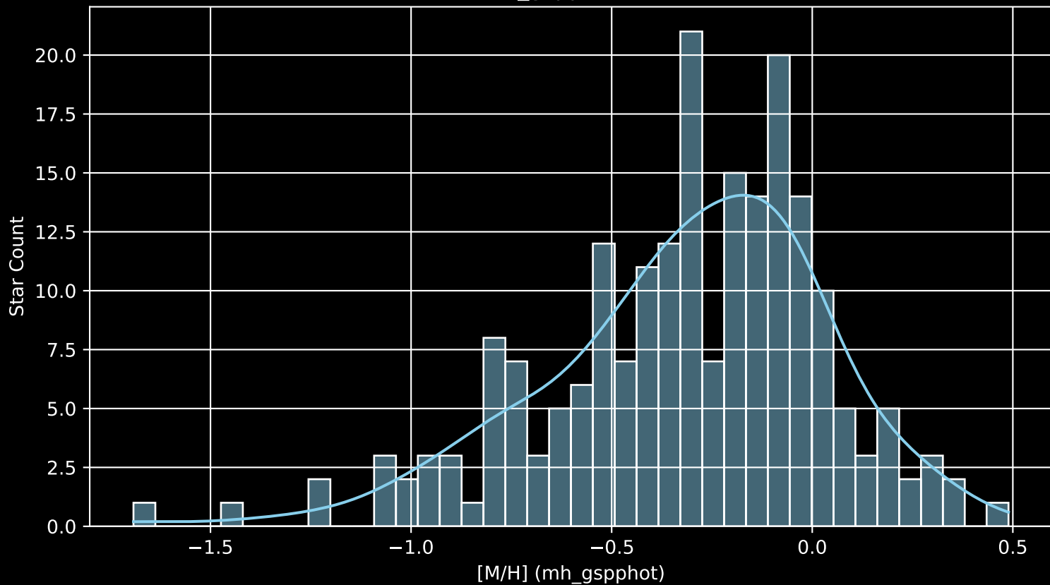
APOGEE DR17 Field: [284-39 [M/H] (mh_gspphot) (n= 209)
