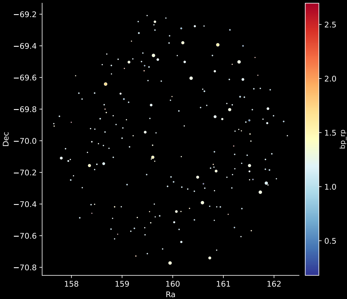
APOGEE DR17 Field: [284-39] Stars: 209
