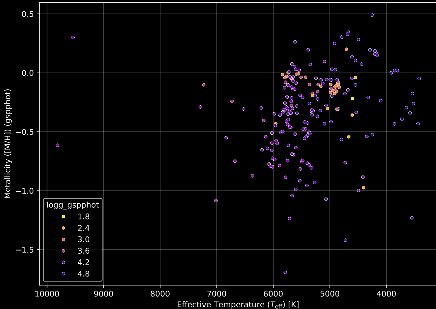
APOGEE DR17 Field: [284-39] Stellar Population Parameters (n= 209)
